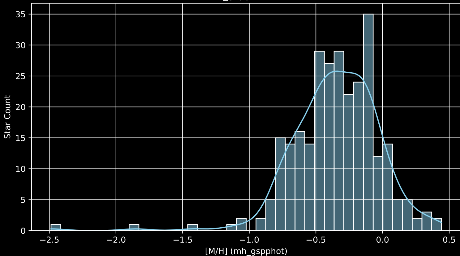
GALAH DR4 Field: [633] [M/H] (mh_gspphot) (n= 281)
