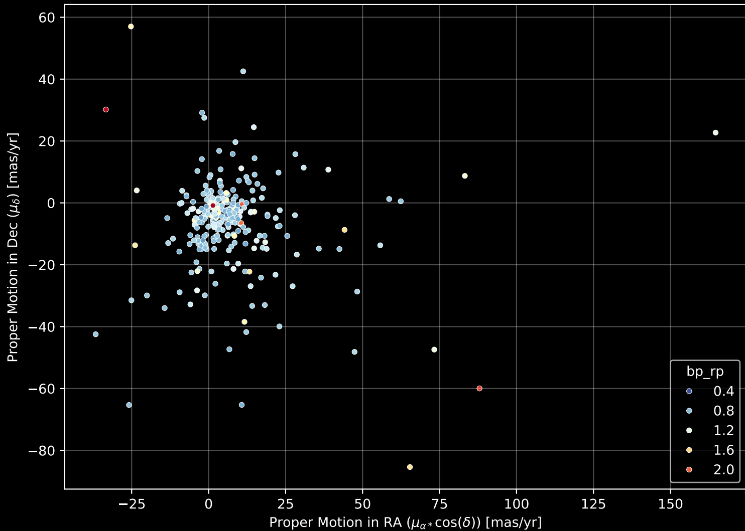
GALAH DR4 Field: [633] Proper Motion Diagram (n= 283)
