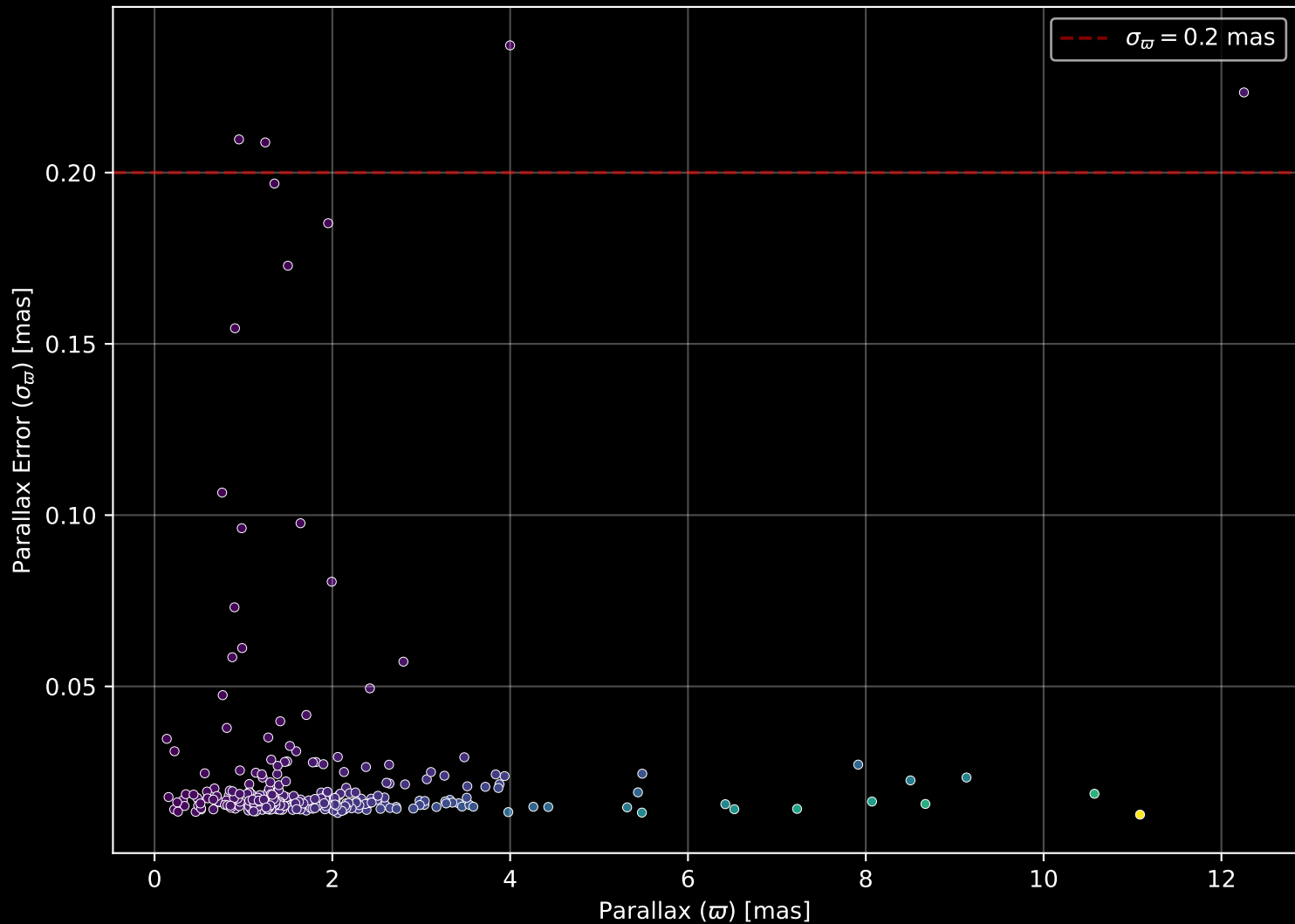
GALAH DR4 Field: [633] Parallax Quality (n= 283)
