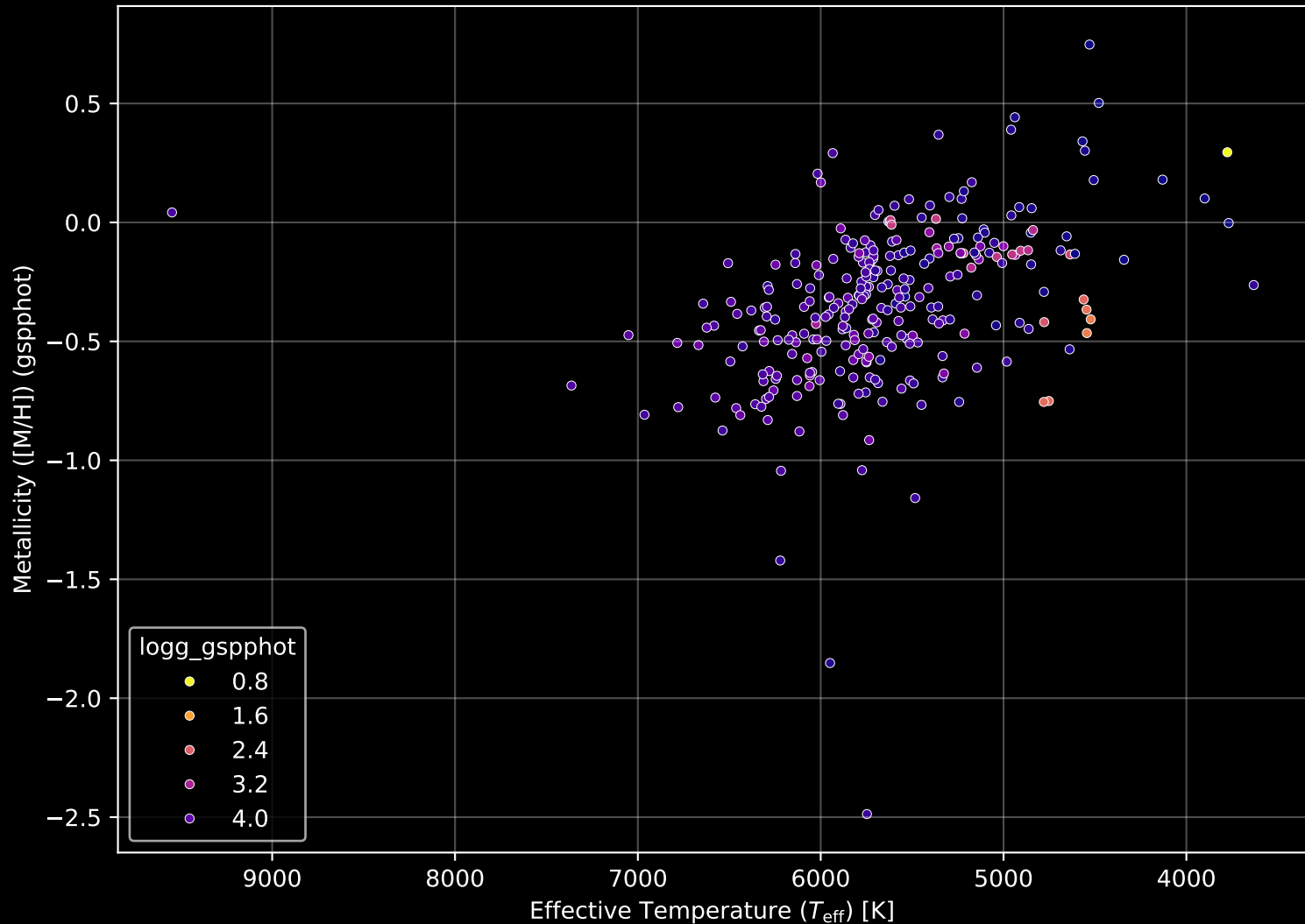
GALAH DR4 Field: [633] Stellar Population Parameters (n= 283)
